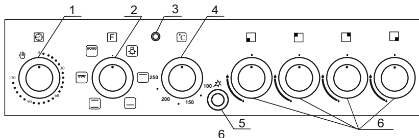
Панель управления плит моделей 606040.01гэ
